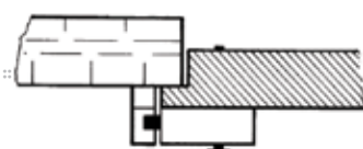
Tür mit Überschlag
